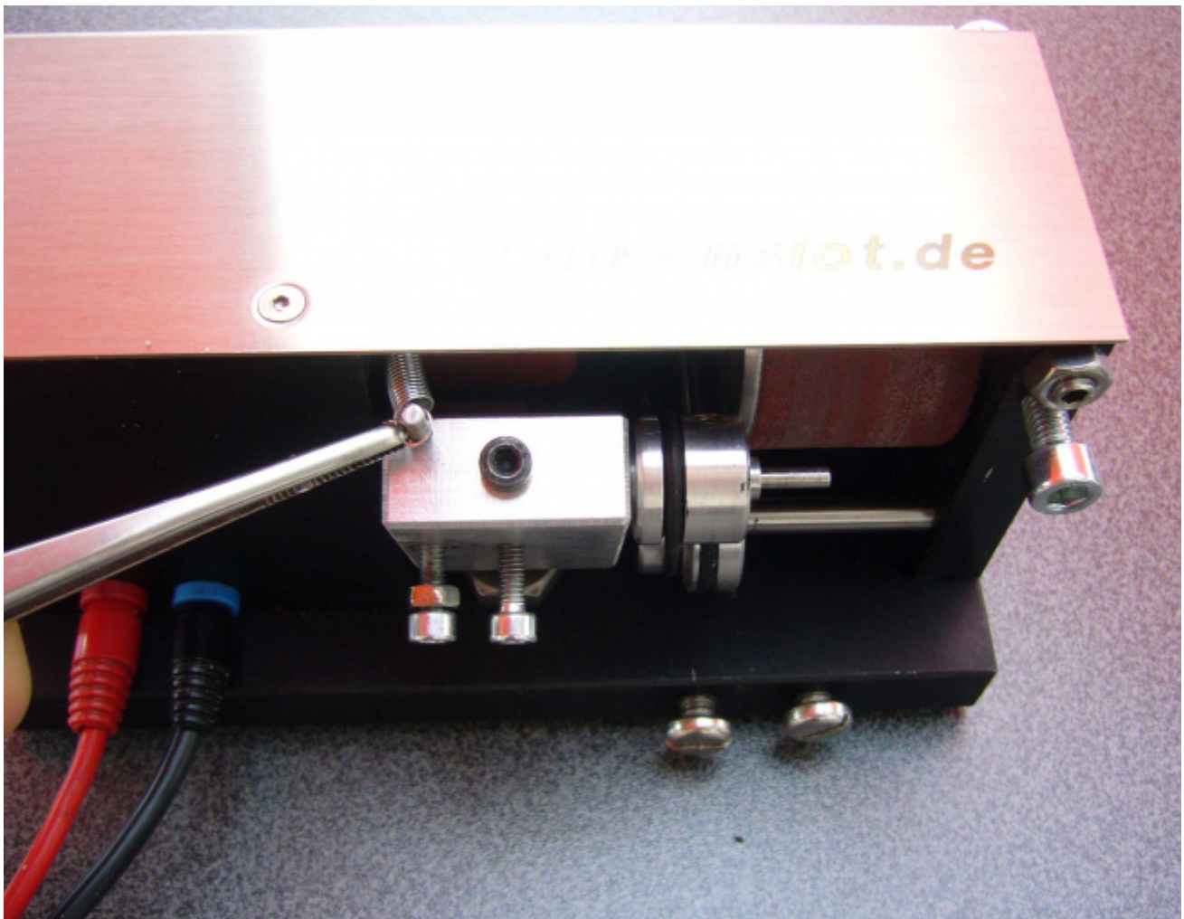
Abb. 1: Rückzugfeder aushängen
